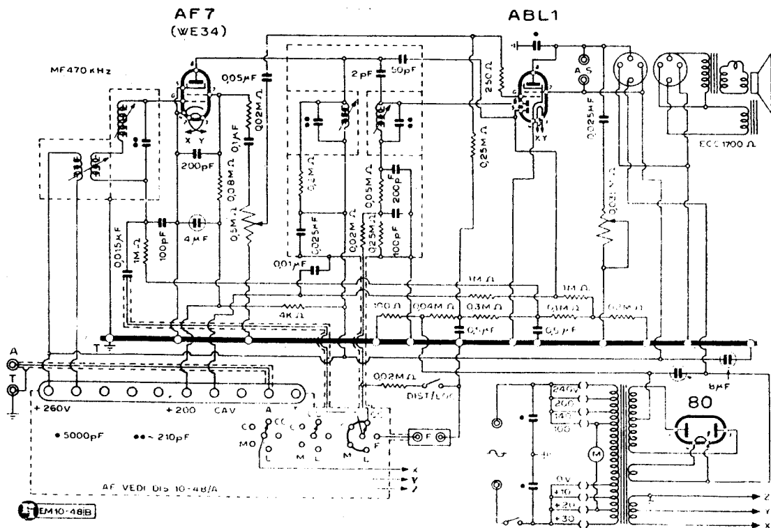
F.I.M.I. - MODD. PHONOLA « 505 » « 506 » - PARTE MF - RIV - BF - ALIM.
