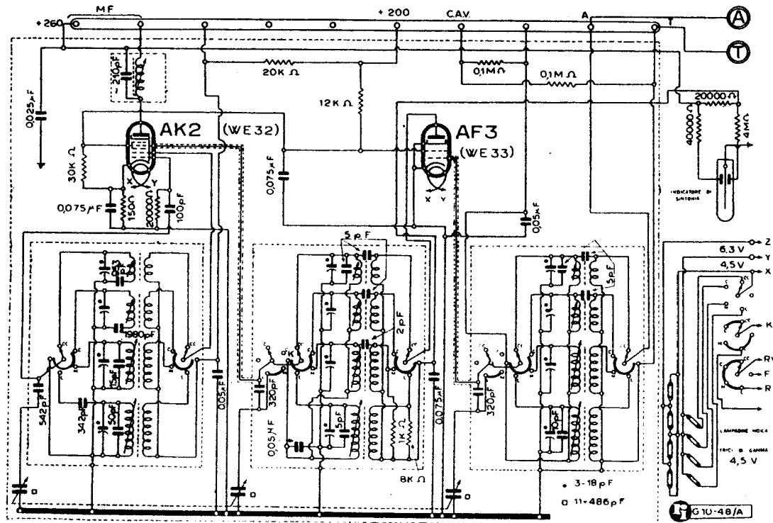
F.I.M.I. - MODD. PHONOLA « 505 » « 506 » - PARTE AF - CONV.
